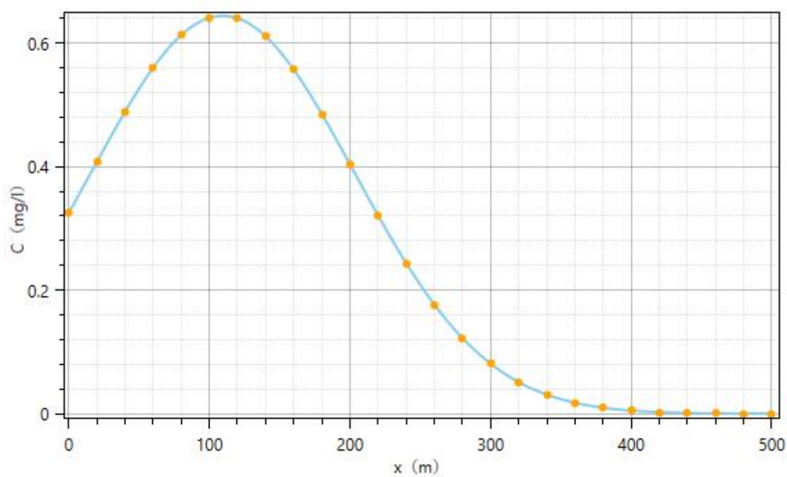
图5.3-14 氨氮运移30a预测结果
