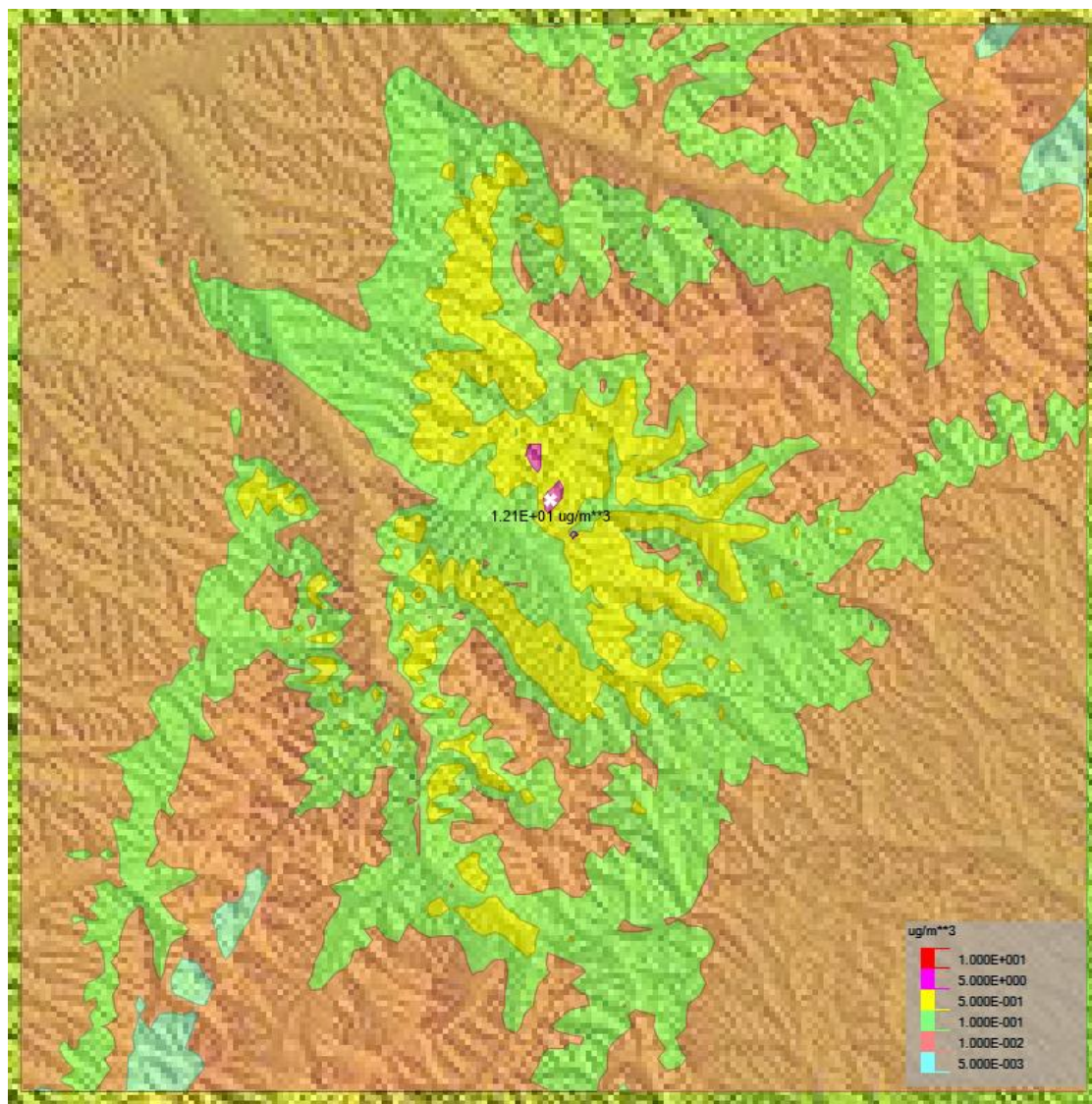
图 5.1-3b 正常工况下 SO 2 最大 24h 平均浓度分布图（单位：μg/m³）
