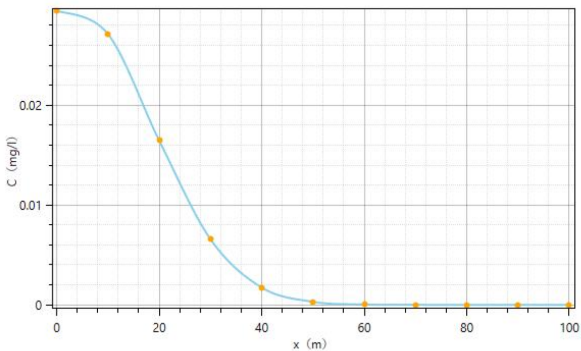
图 5.3-9 铅运移 100d 预测结果
