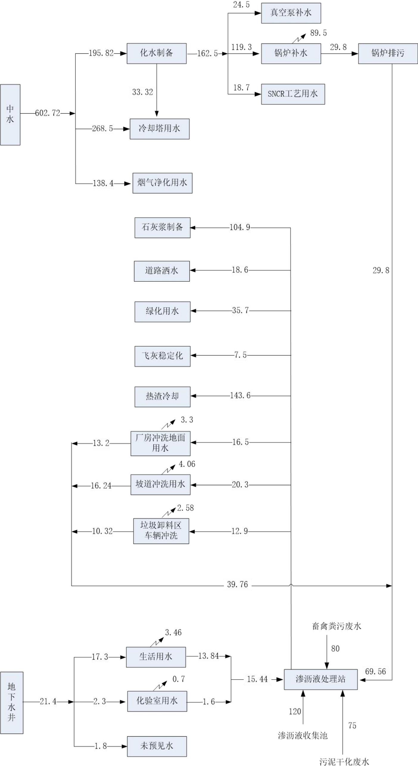
图 3.1-2 非采暖期水平衡图 (m³/d)
