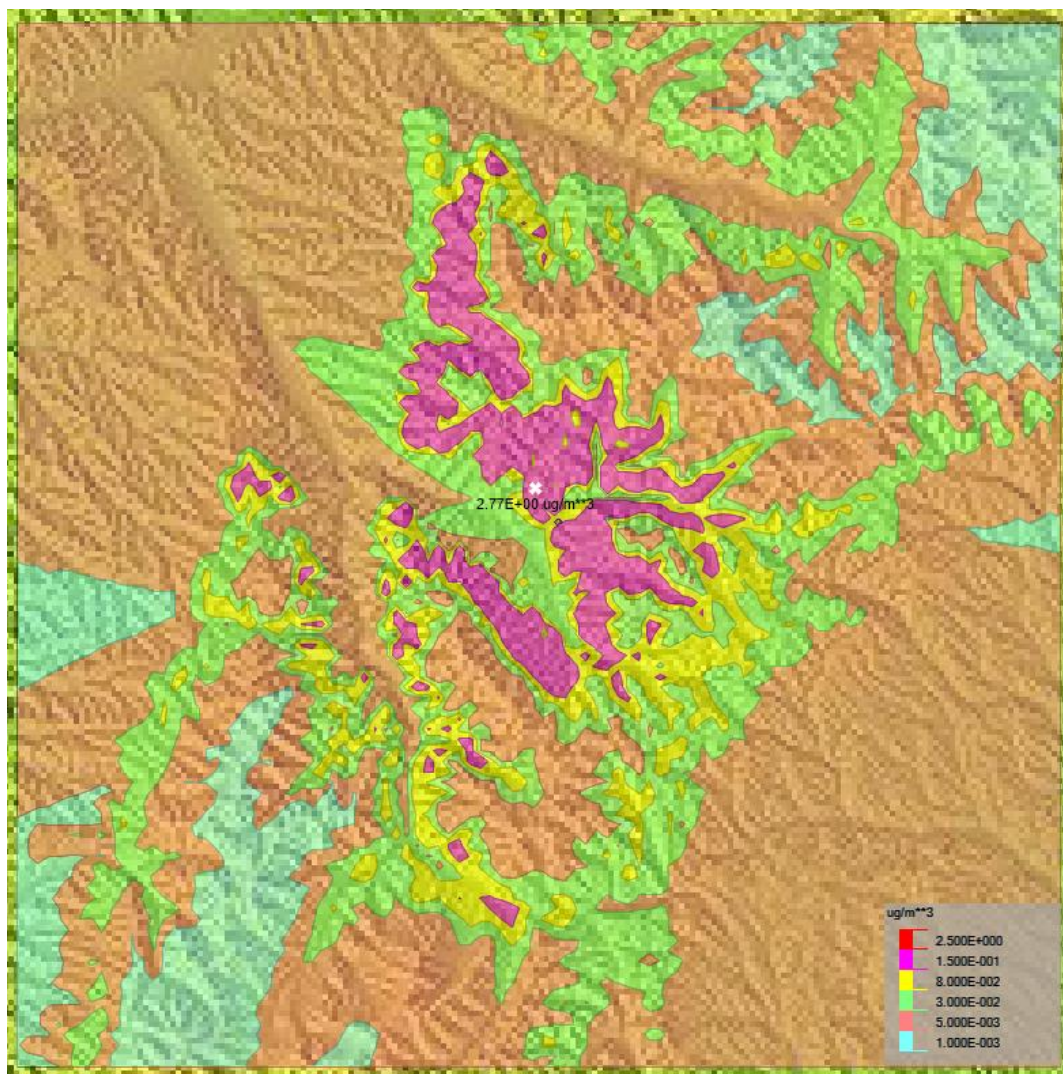
图 5.1-7b 正常工况下 HCl 最大 24h 平均浓度分布图（单位： \mu\text{g}/\text{m}^3 ）
