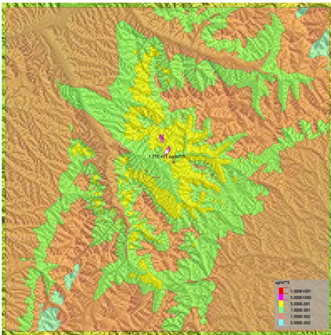
图 5.1-3b 正常工况下 SO 2 最大 24h 平均浓度分布图（单位：μg/m 3 ）
