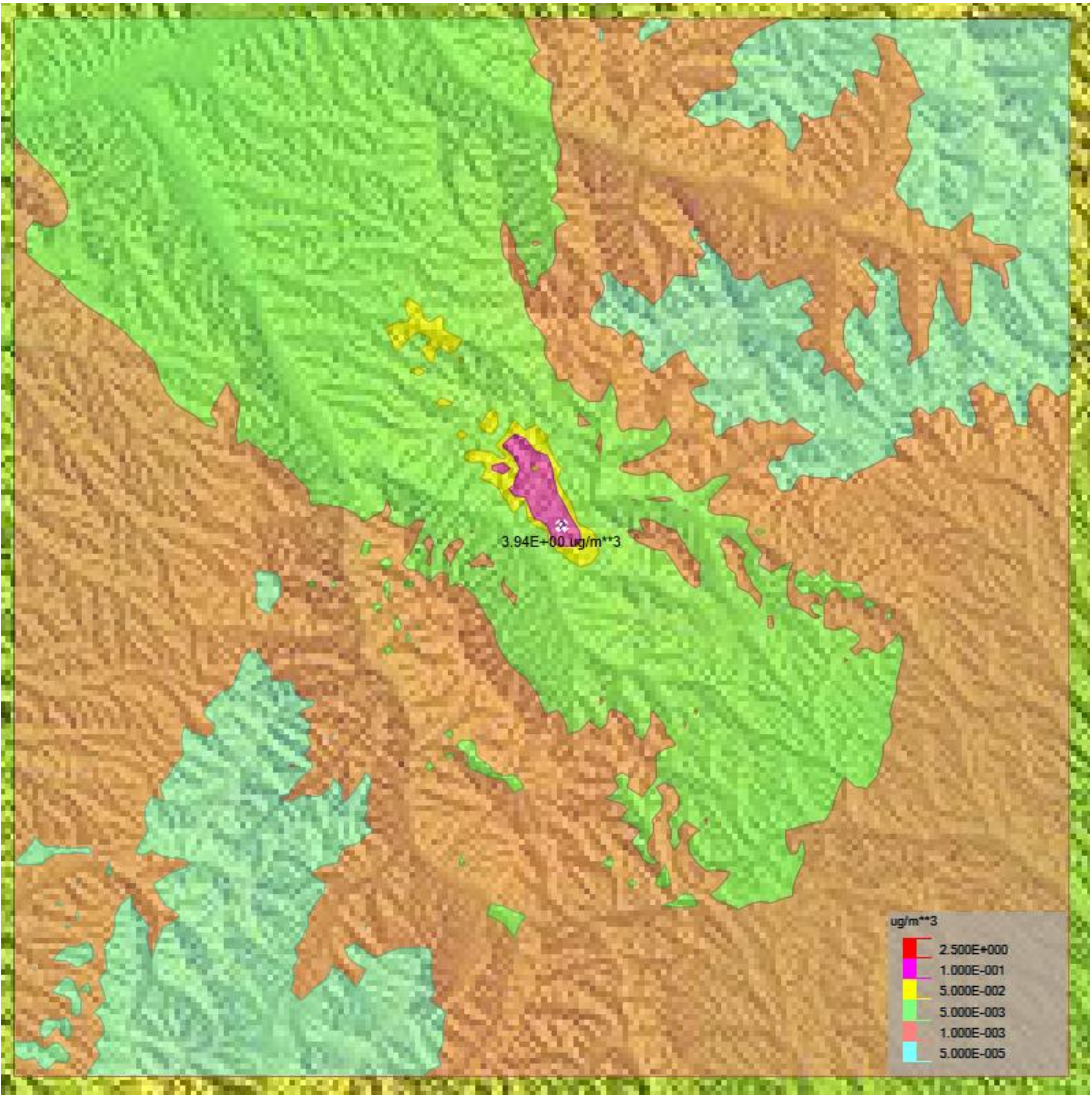
图 5.1-5b 正常工况下 PM 10 年平均浓度分布图（单位：µg/m 3 ）
