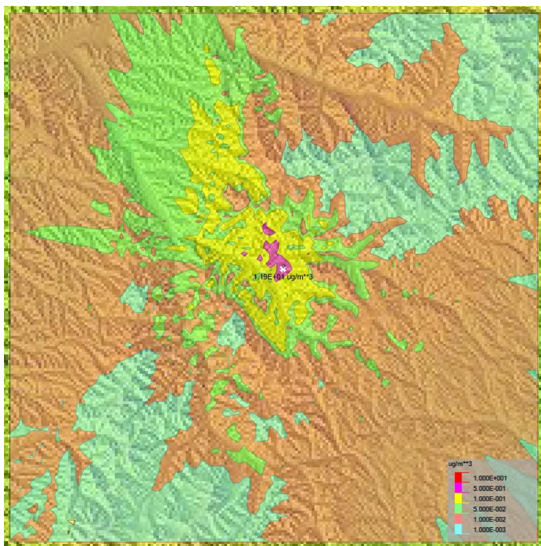
图 5.1-6a 正常工况下 PM 2.5 最大 24h 平均浓度分布图 (单位: \mu\text{g}/\text{m}^3 )
