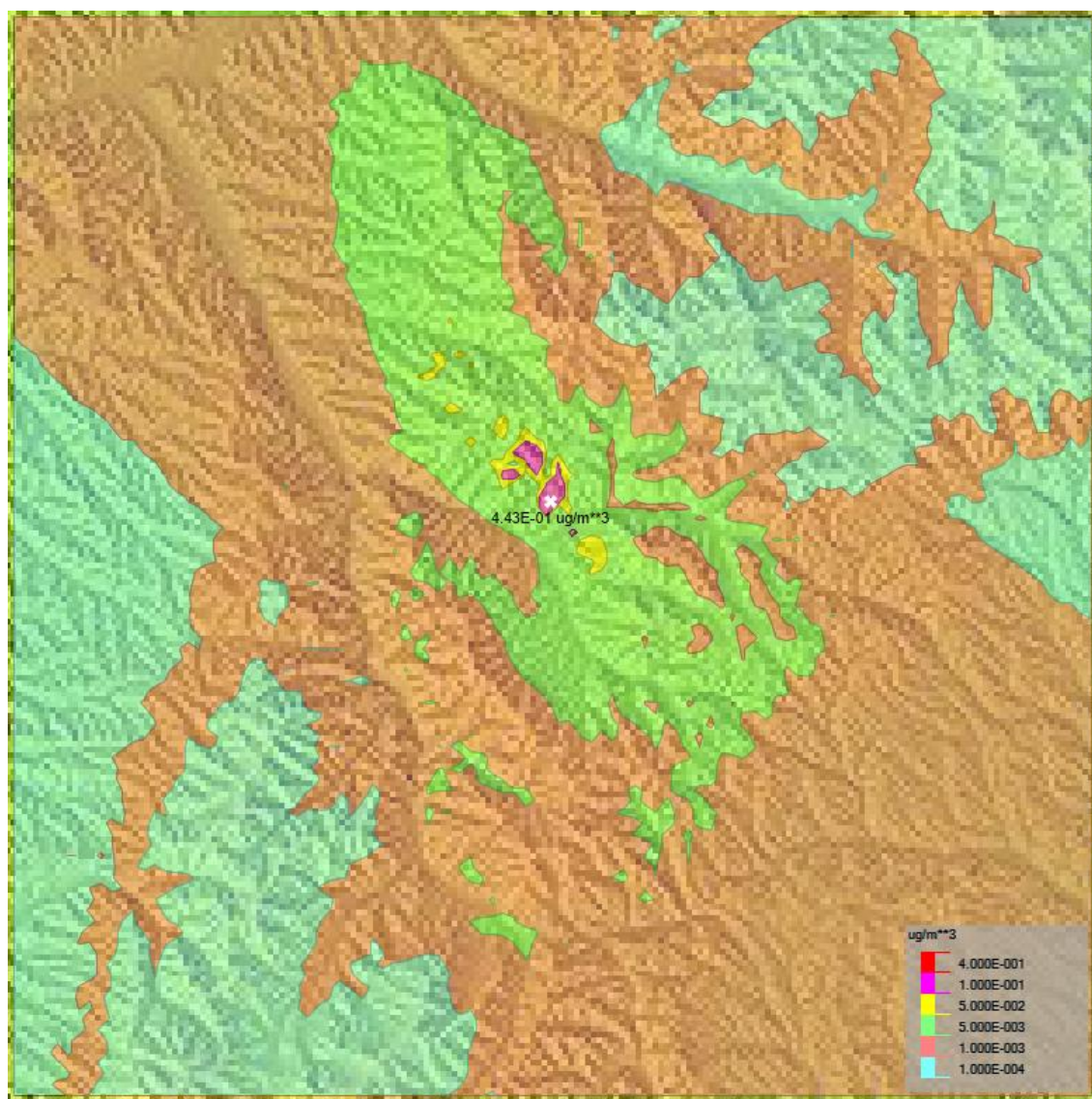
图 5.1-11 正常工况下 H 2 S 最大 1h 平均浓度分布图（单位：μg/m 3 ）
